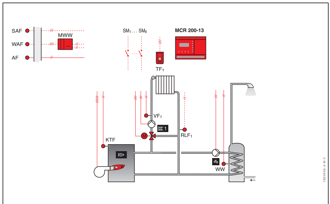
Anlage mit 3-Wege-Mischer
