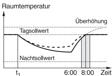
Außentemperatur ca. +5°C (temperaturvariable Aufheizung, Aufheizzeit = 2 h)
