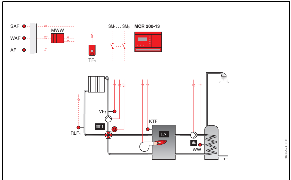
Anlage mit 4-Wege-Mischer
