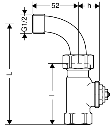
Abb. 10. Durchgang mit Bogentülle
